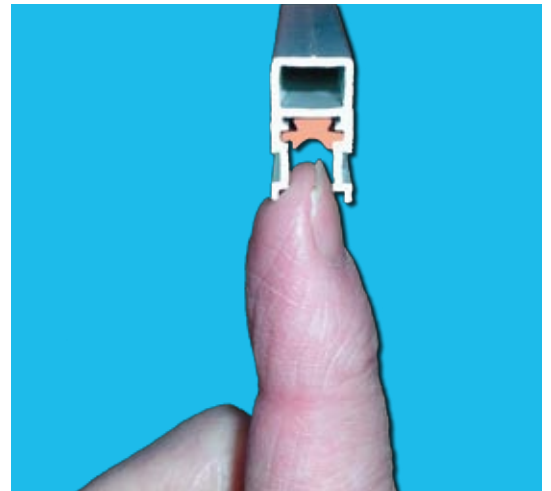
Fig. 1 - Protection contre le toucher au conducteur.
