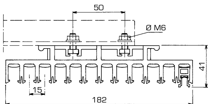
Fig. 3 - Suspension d'une barrette à griffes jusqu'à 12 conducteurs.
